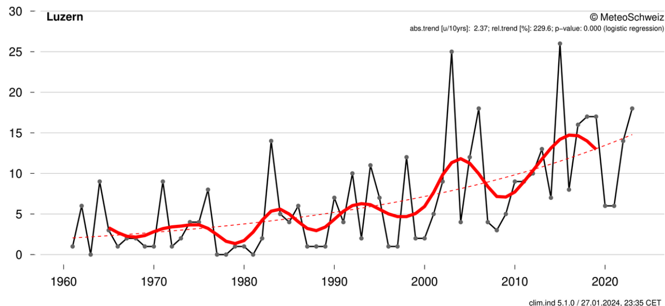
Hitzetage [Tmax >= 30°C] (Tage) Kalenderjahr (Jan.–Dez.) 1961–2023
